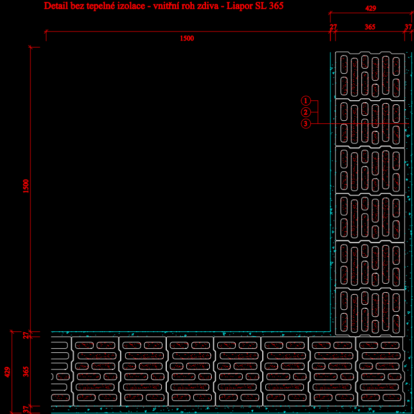
Detail bez tepelné izolace - vnitřní roh zdíva - Liapor SL 365
