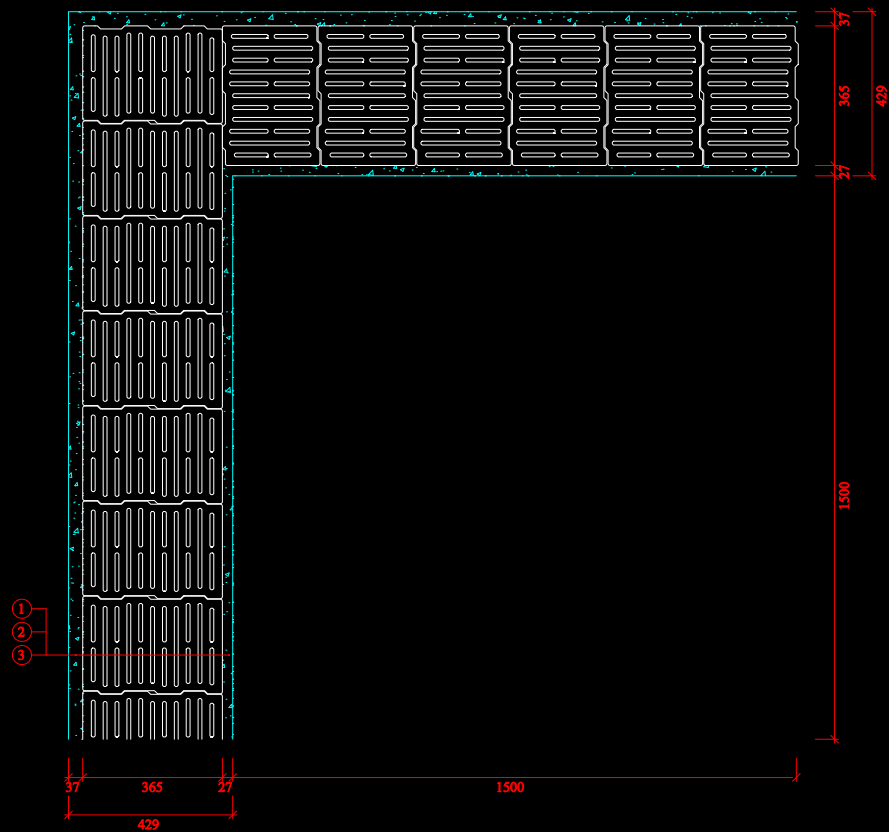
Detail bez tepelné izolace - vnější roh zdiva - Liatherm 365
