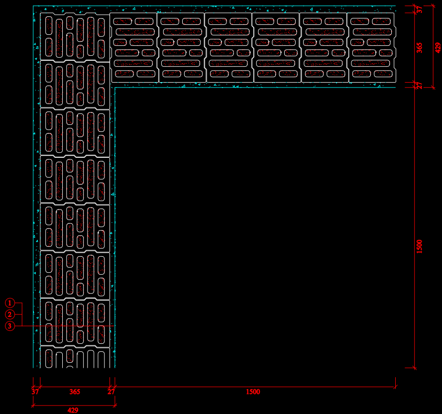
Detail bez tepelné izolace - vnější roh zdiva - Liapor SL 365
