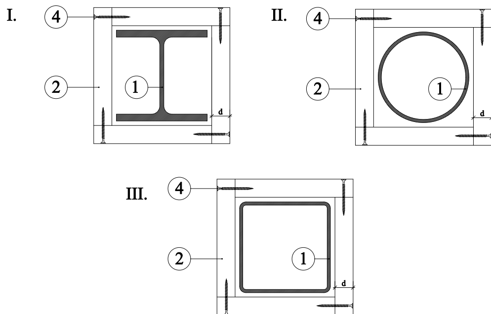
Detail A - příklady provedení
