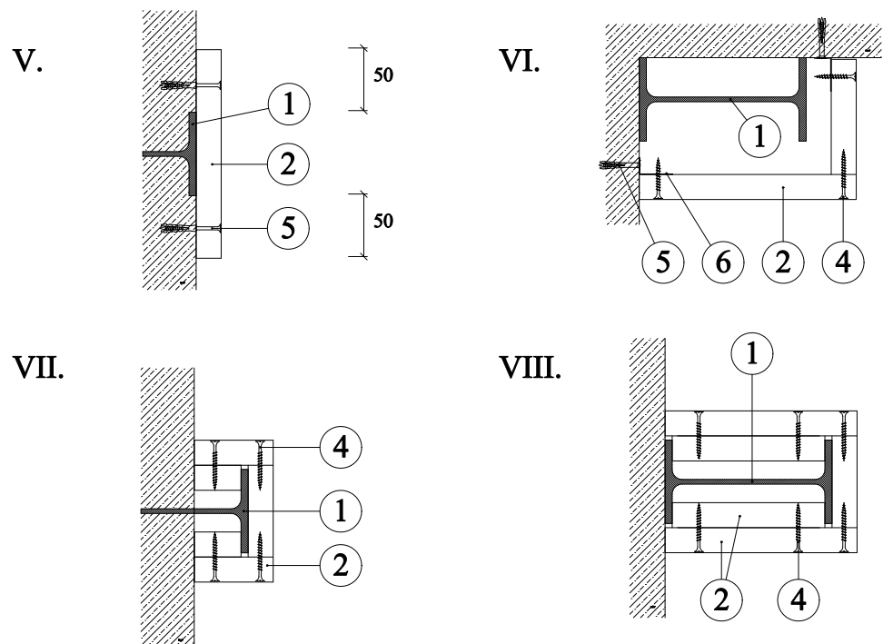
Detail B – jedno-, dvou- a třístranná obložení
